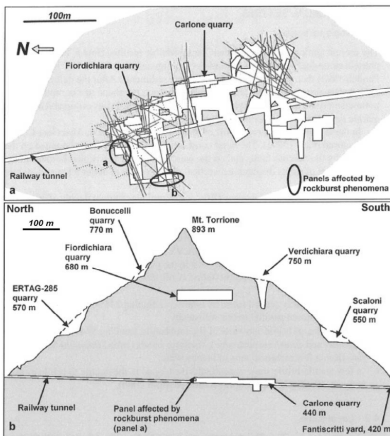
Rys. 1. Lokalizacja kopalni Carlone w obrębie góry Torrione a) plan wyrobisk ze śladami występujących spekań (nieregularne kreskowania), b) przekrój poprzeczny wzdłuż tunelu nieczynnej kolejki (Coli 2001)
