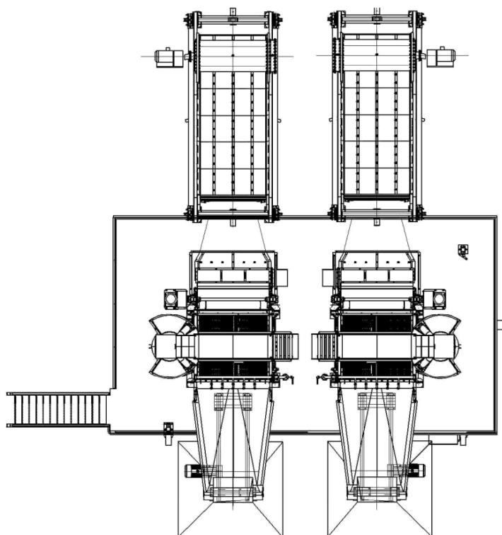
Rys. 5. Koncepcja układu do oczyszczania kruszywa z ziaren o wysokiej gęstości (Kowol 2013)
