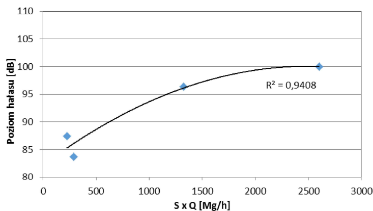
Rys. 5. Poziom hałasu na łączny efekt wydajności i stopnia rozdrobnienia Fig. 5. Noise level per cumulative effect of comminution and throughput
