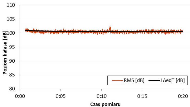
Rys. 2. Zarejestrowany poziom hałasu dla kruszarki walcowej Fig. 2. Noise level for roller crusher
