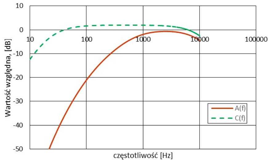
Rys. 1. Przebieg krzywych korekcyjnych A i C Fig. 1. Correction curves A and C type
